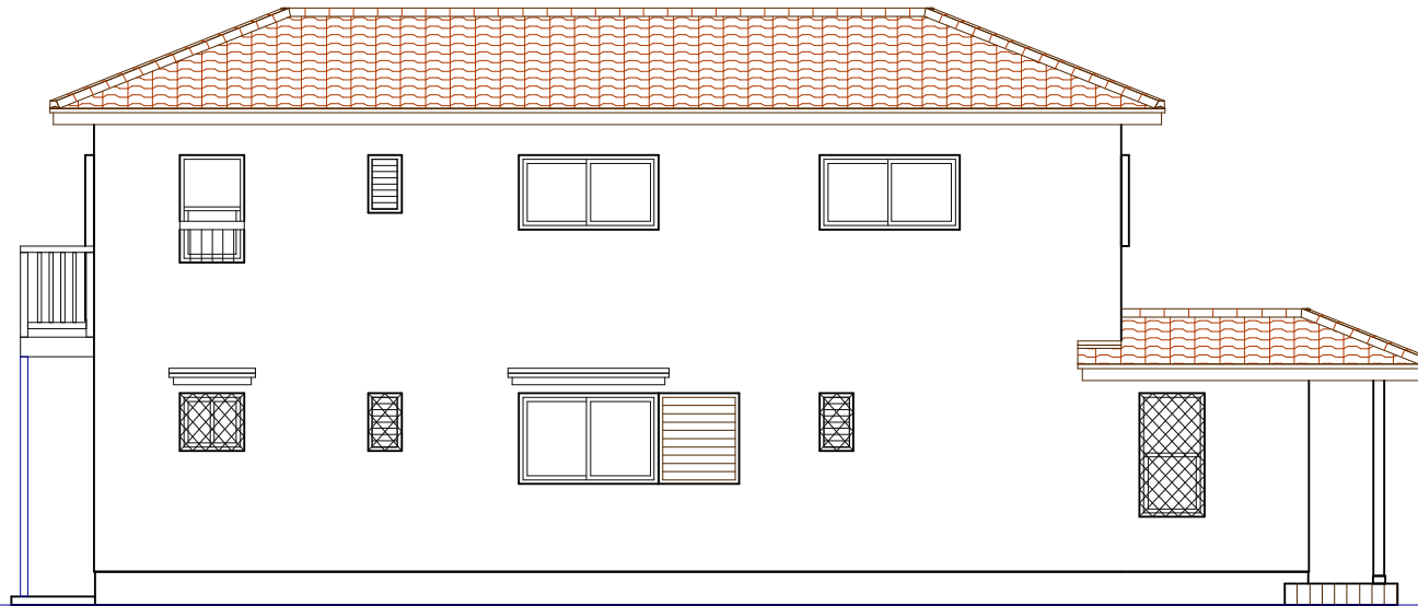
北側立面図
