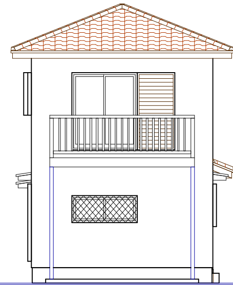
東側立面図
