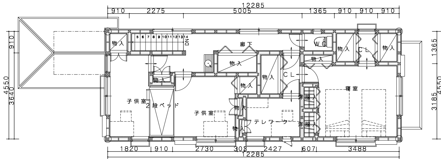
2階平面図
