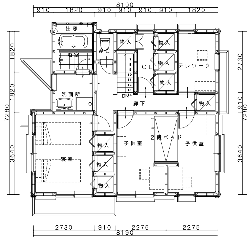
2階平面図
