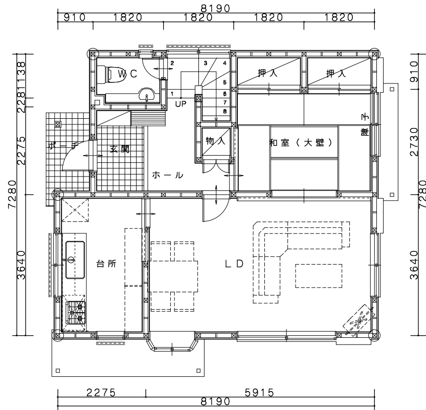
1階平面図
