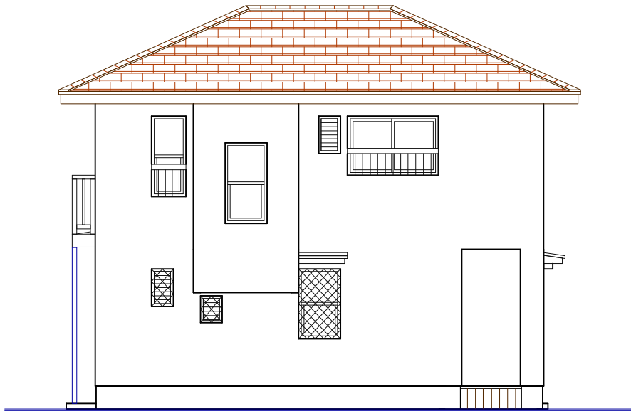
北側立面図
