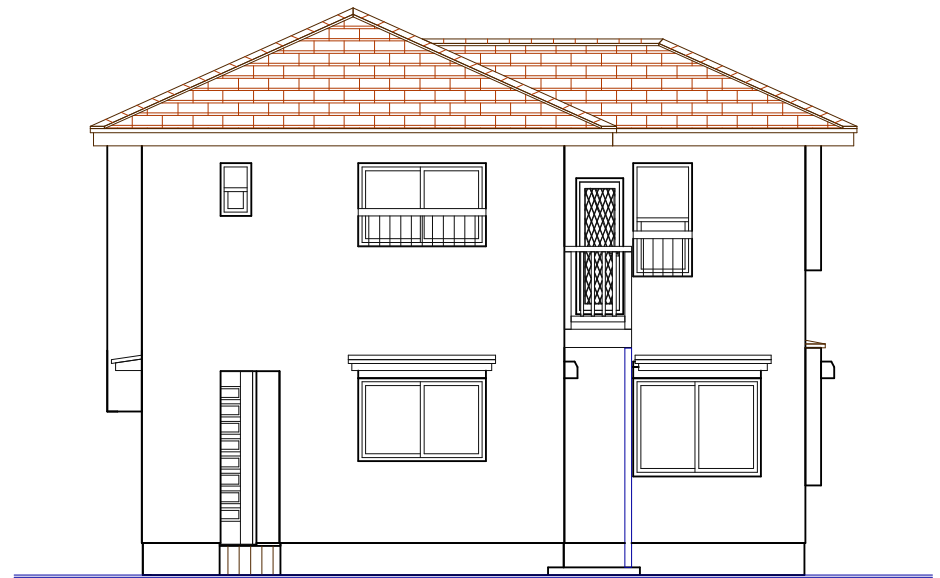
西側立面図
