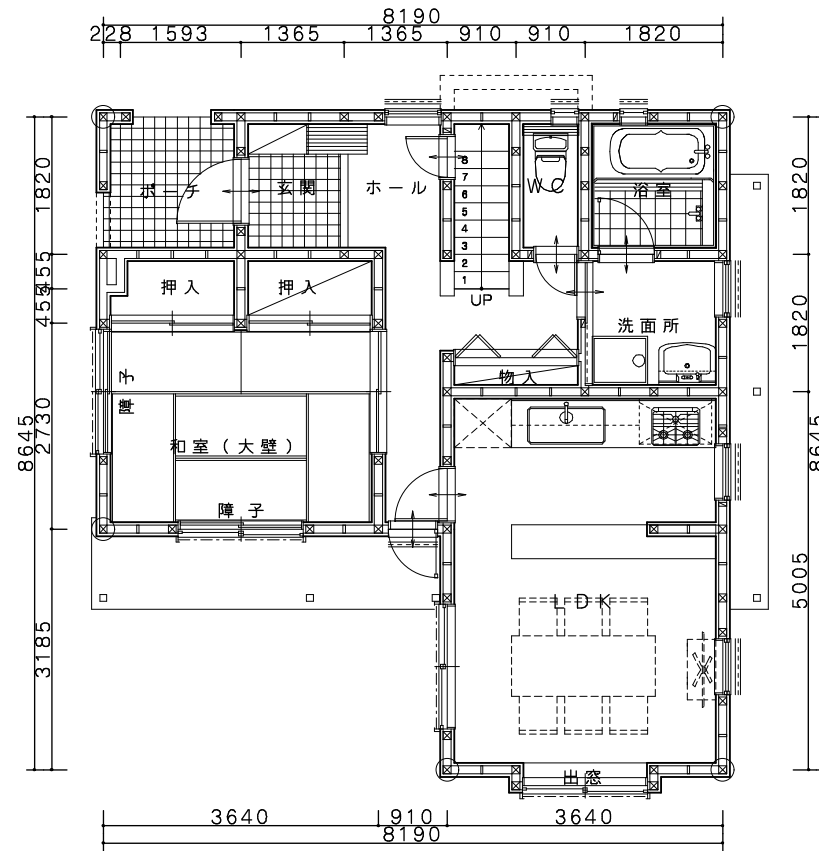
1階平面図
