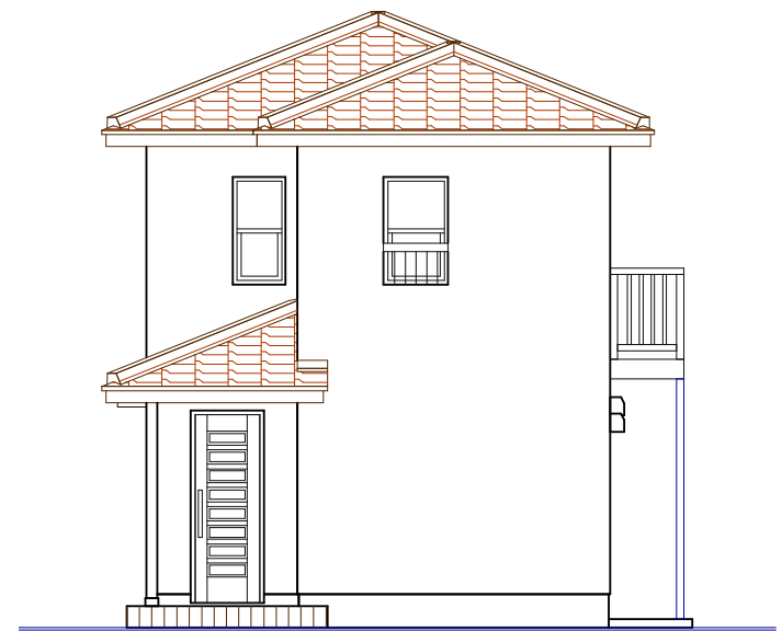
西側立面図
