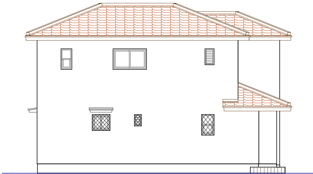
北側立面図
