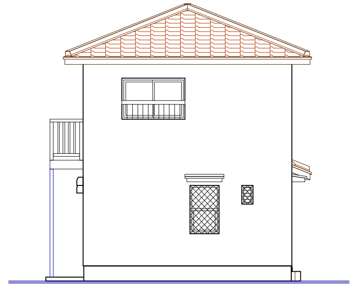
東側立面図
