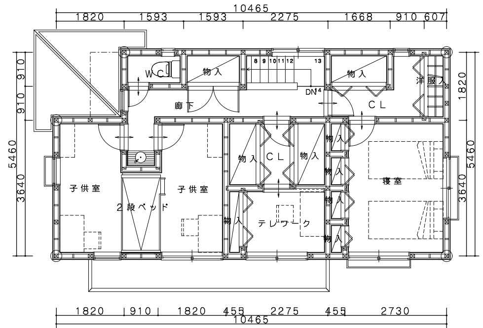
2階平面図
