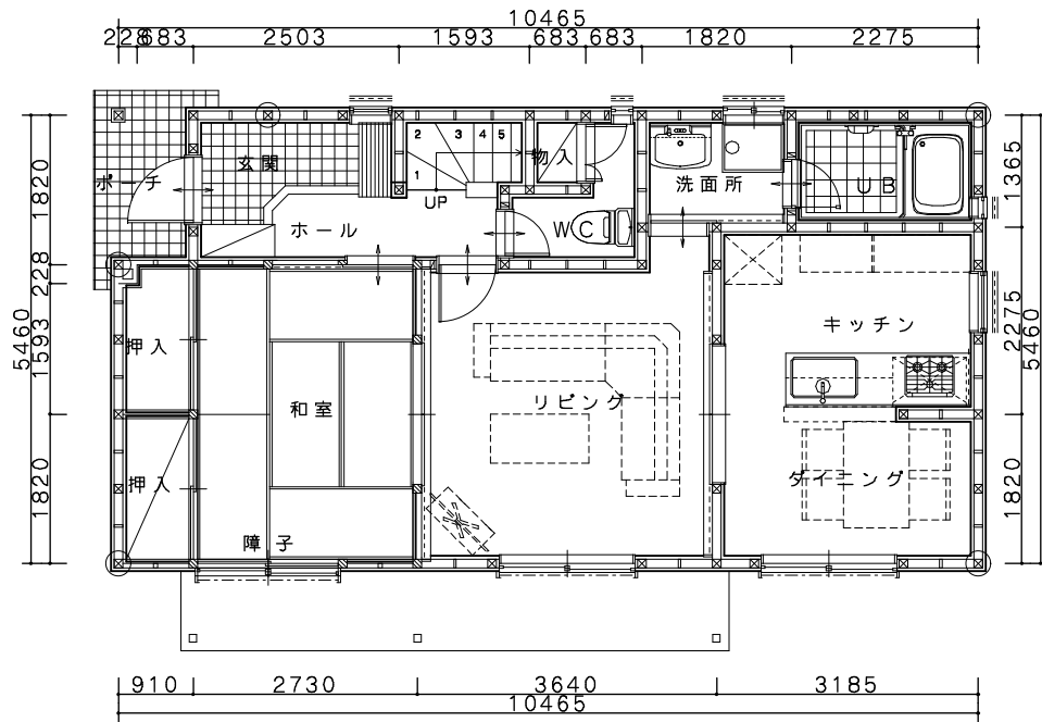
1階平面図
