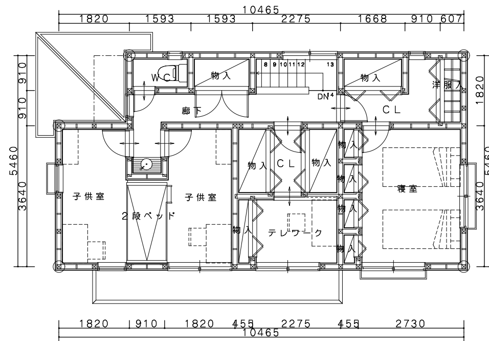
2階平面図
