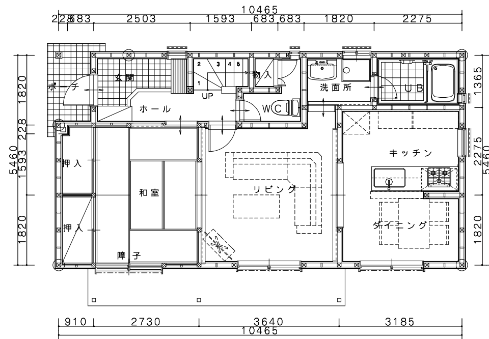
1階平面図
