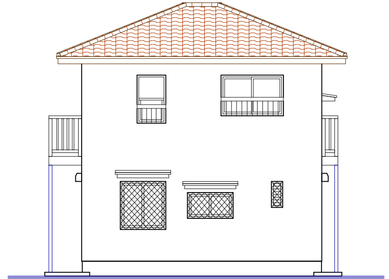
東側立面図
