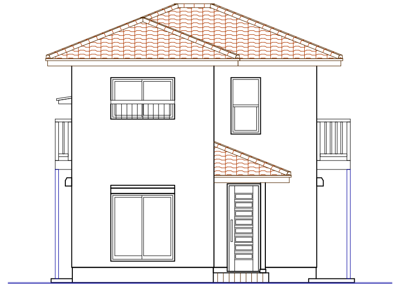
西側立面図
