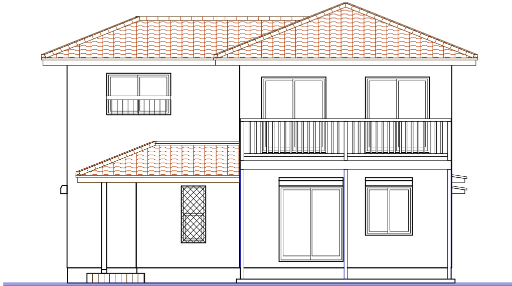
南側立面図
