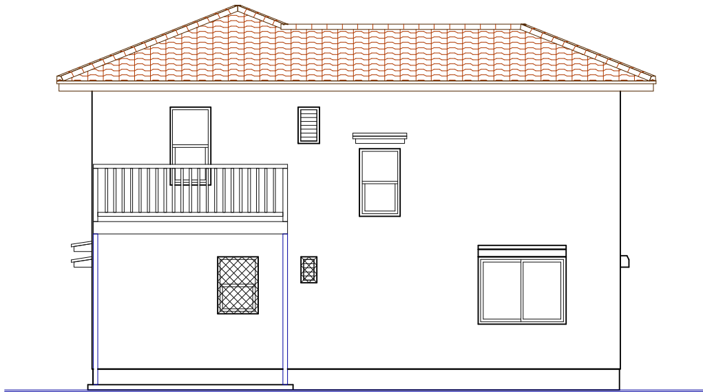
北側立面図
