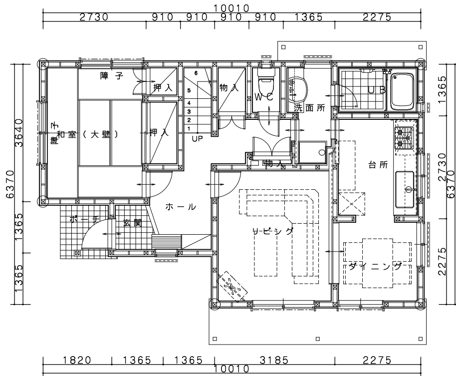
1階平面図
