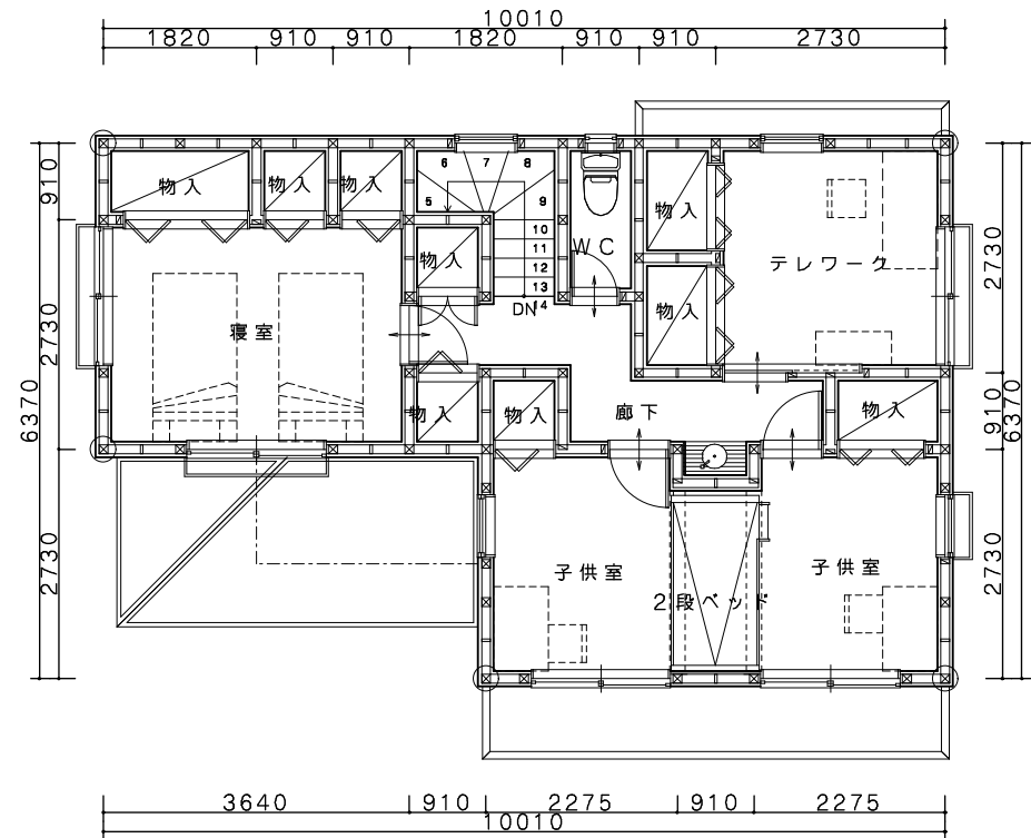
2階平面図
