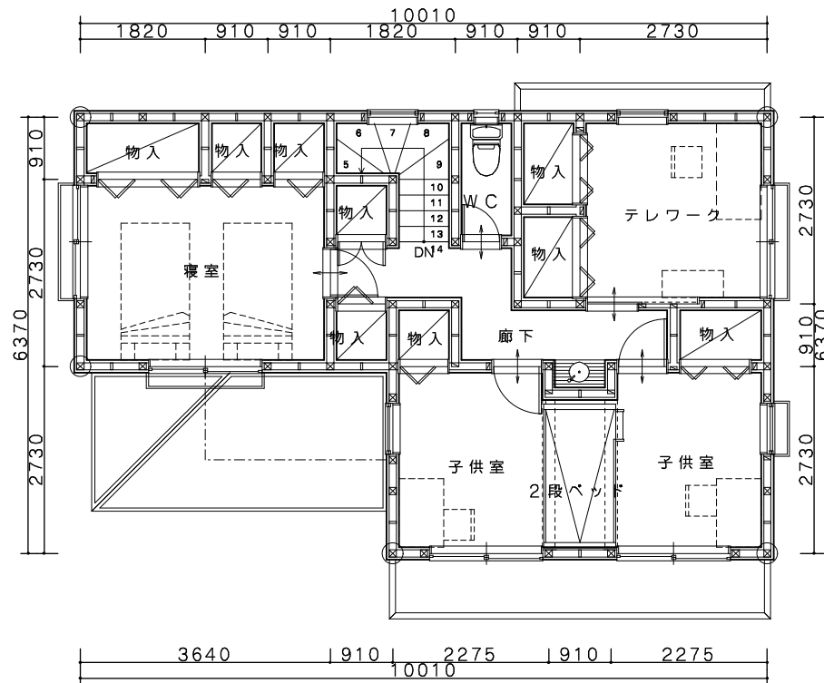
2階平面図
