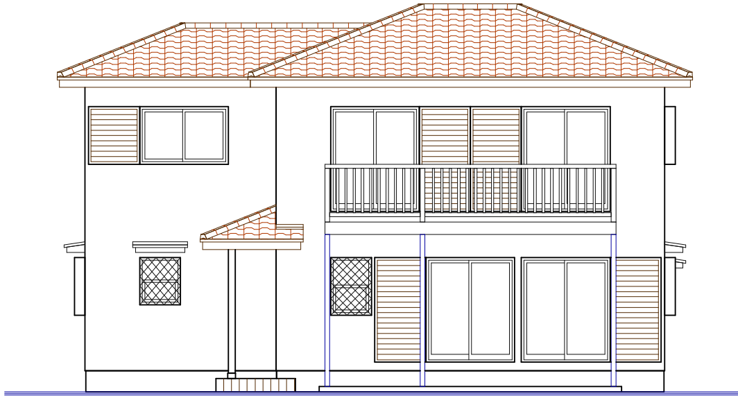
南側立面図
