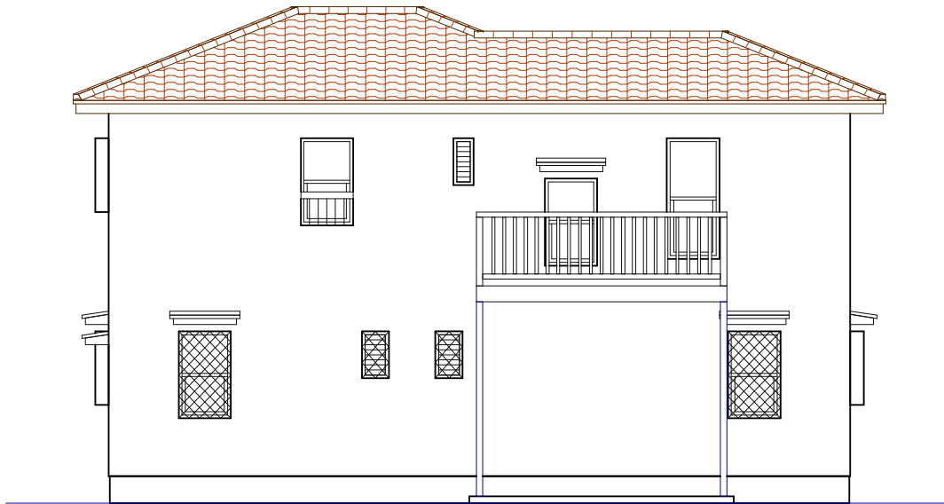
北側立面図
