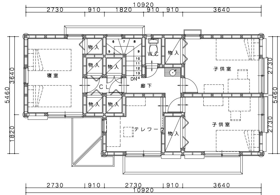
2階平面図
