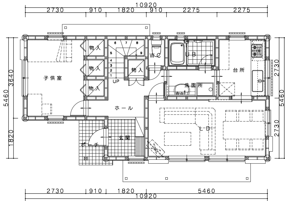
1階平面図
