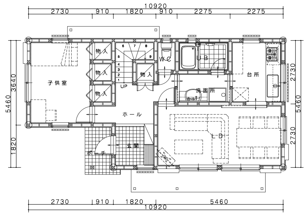
1階平面図
