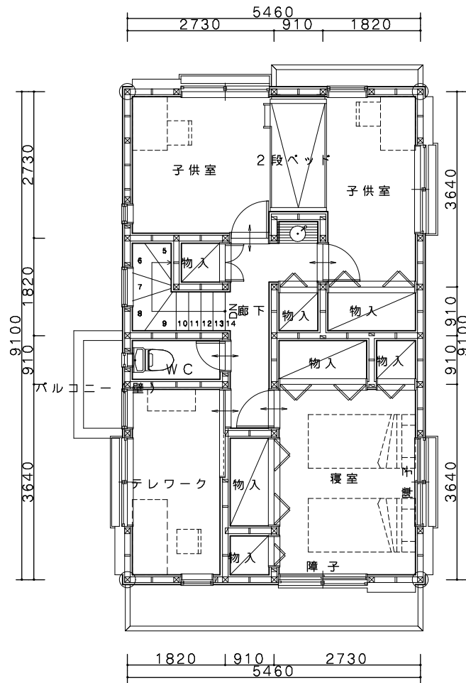
2階平面図
