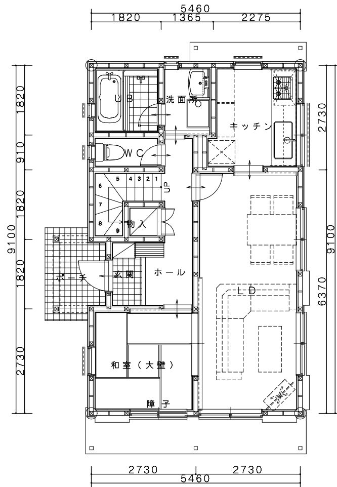
1階平面図
