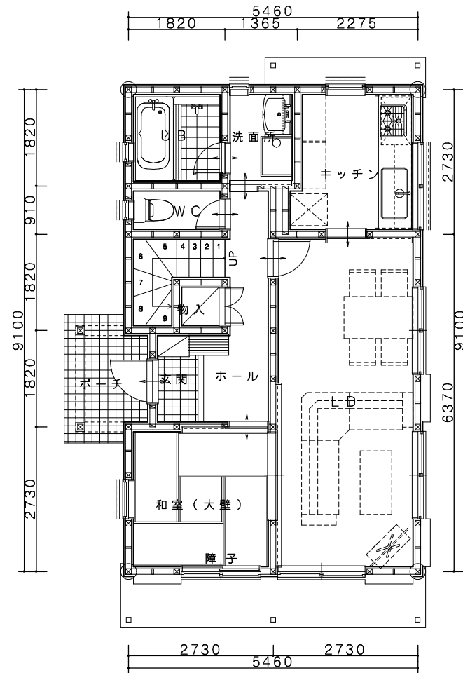
1階平面図
