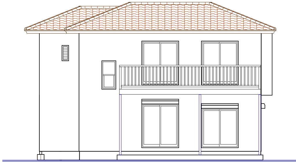
南側立面図
