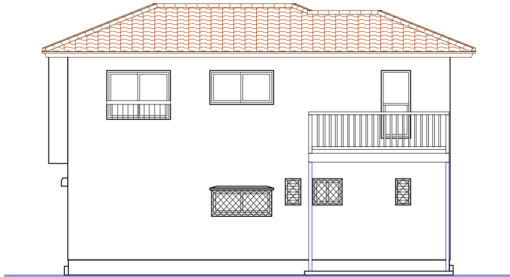
北側立面図
