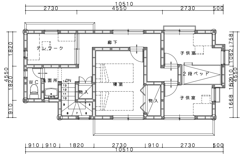
2階平面図
