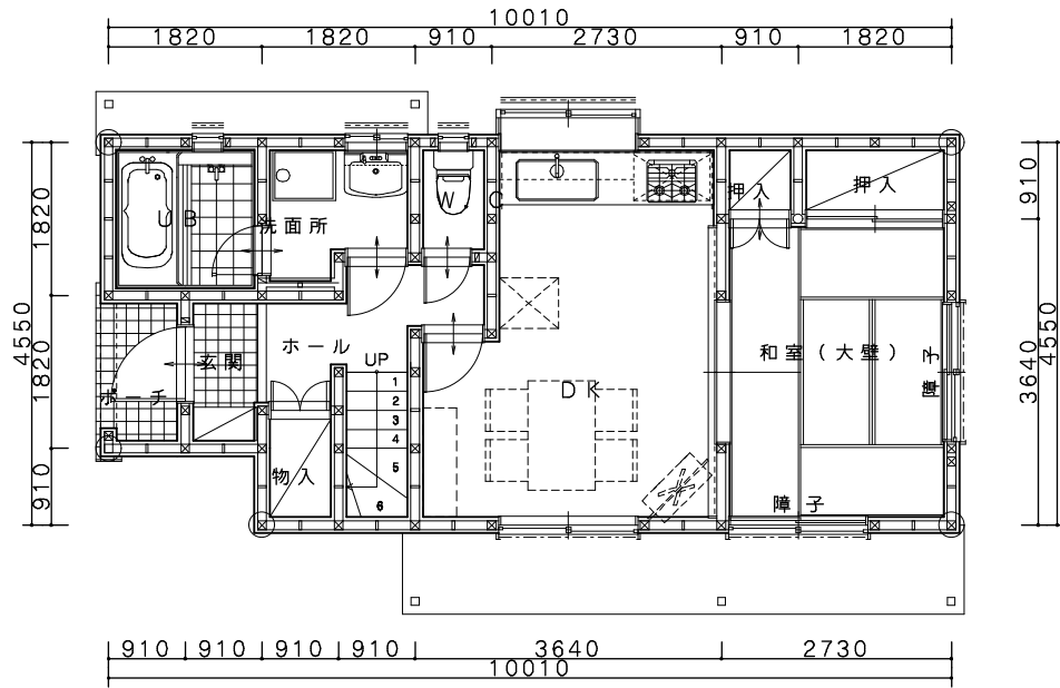
1階平面図
