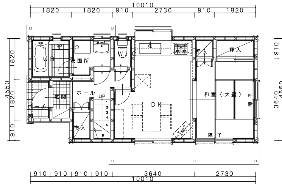
1階平面図
