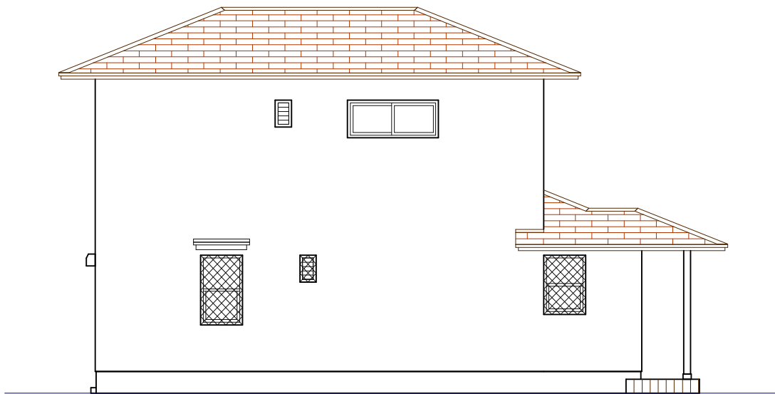
北側立面図
