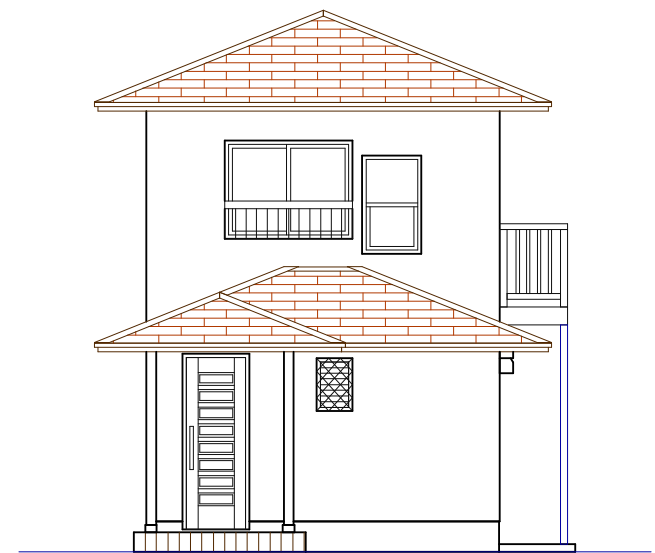
西側立面図
