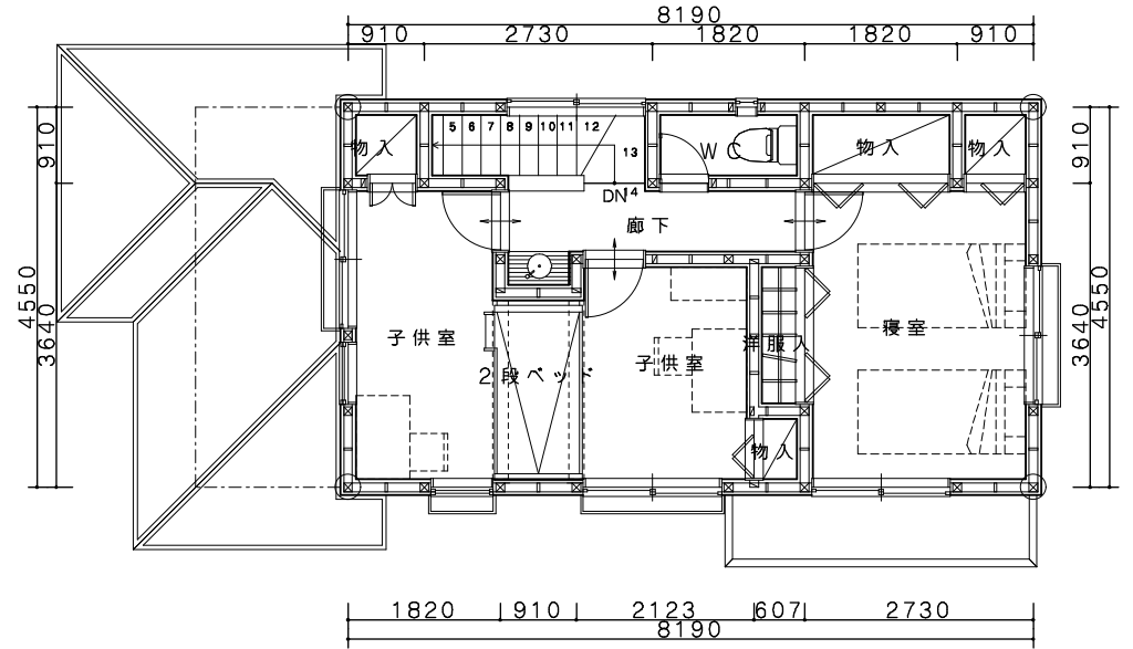
2階平面図
