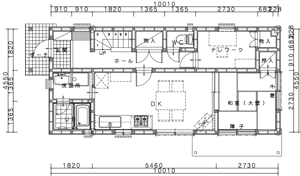
1階平面図
