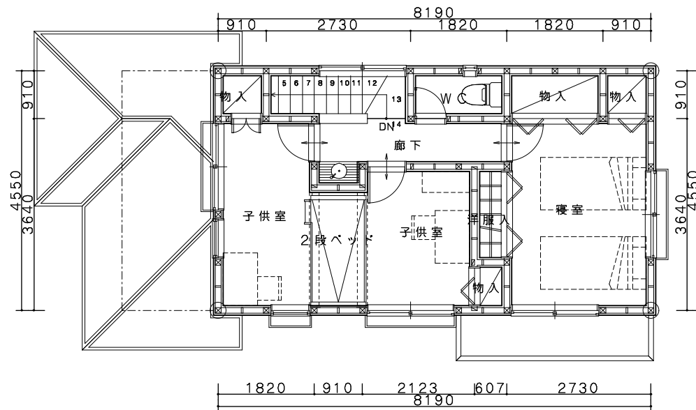
2階平面図
