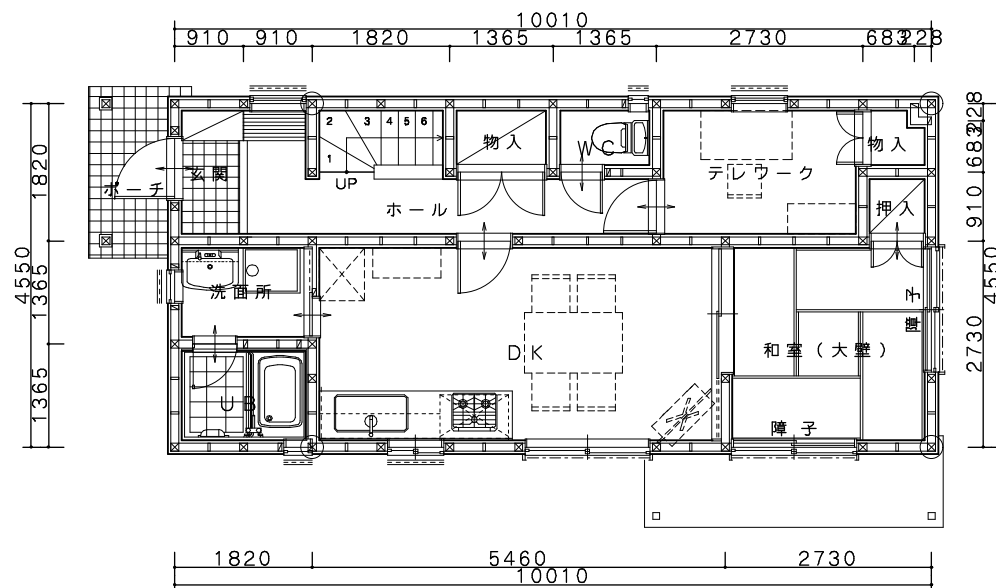
1階平面図
