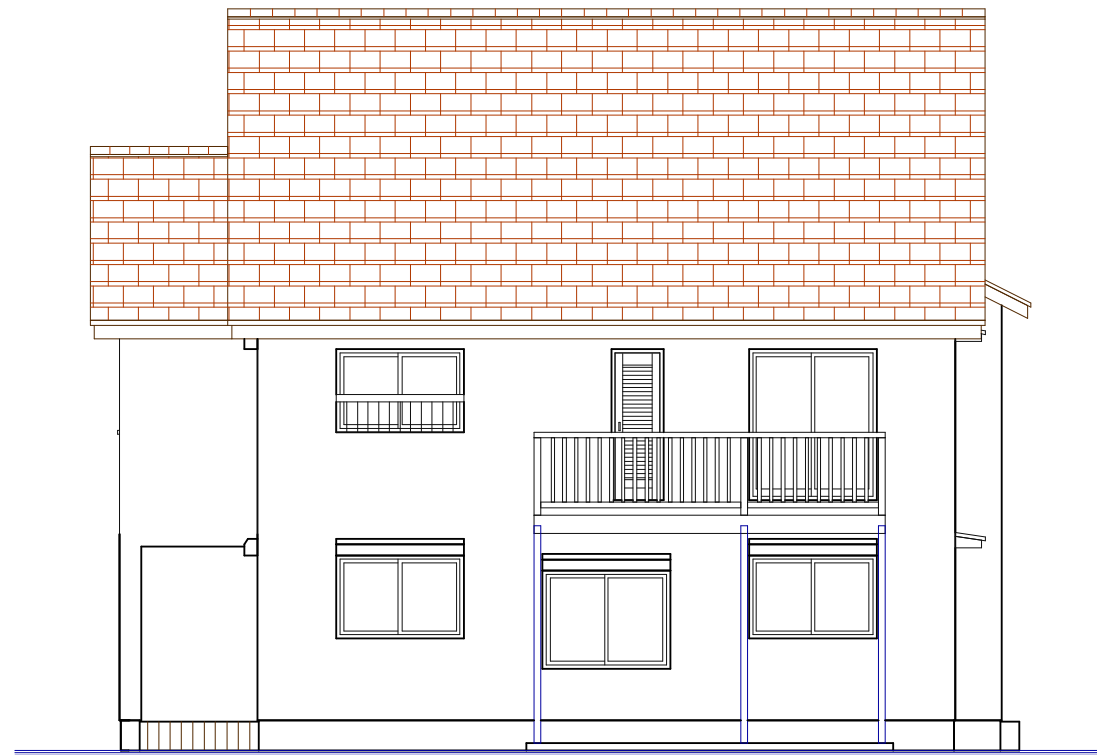
東側立面図
