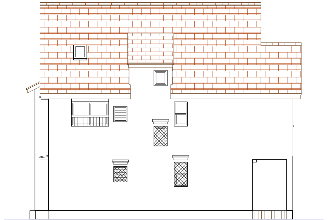
西側立面図
