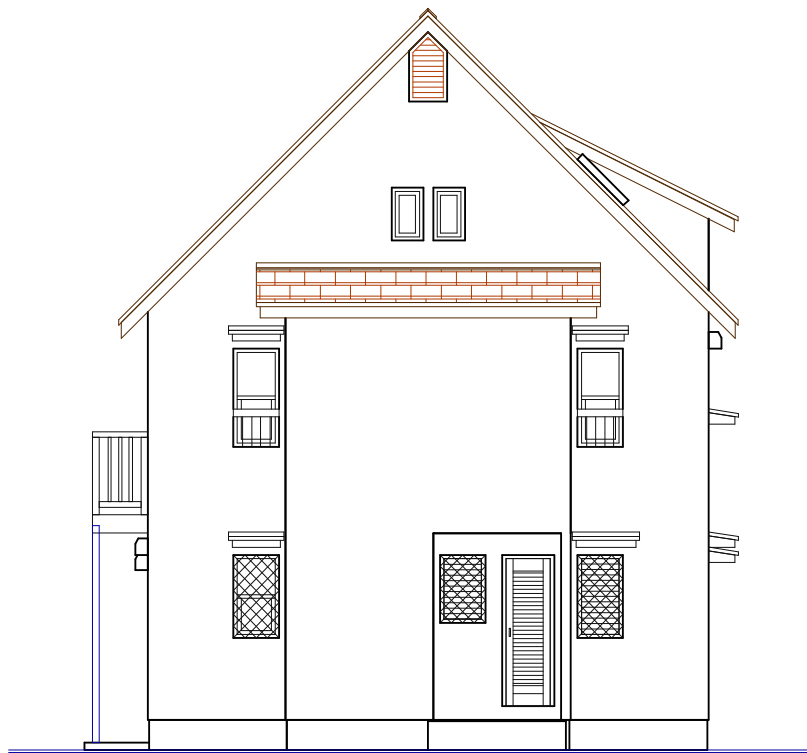
北側立面図
