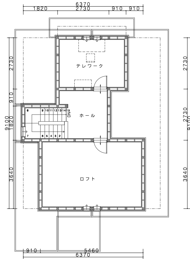
3階平面図
