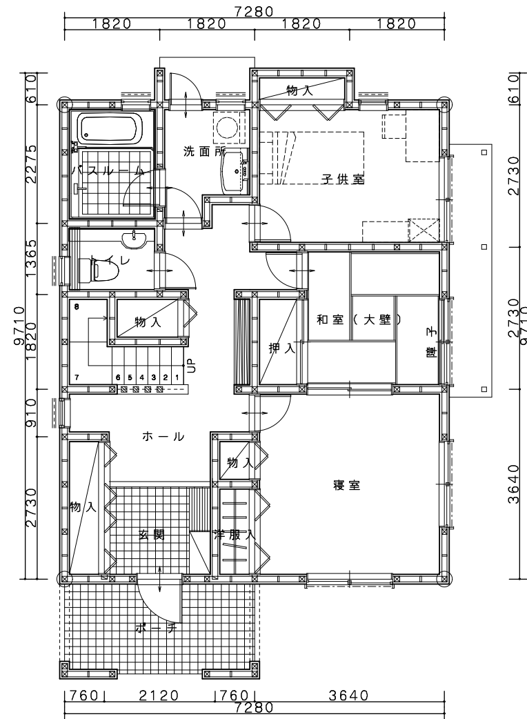
1階平面図
