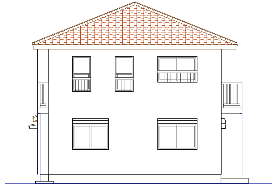
西側立面図
