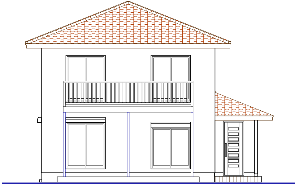
南側立面図
