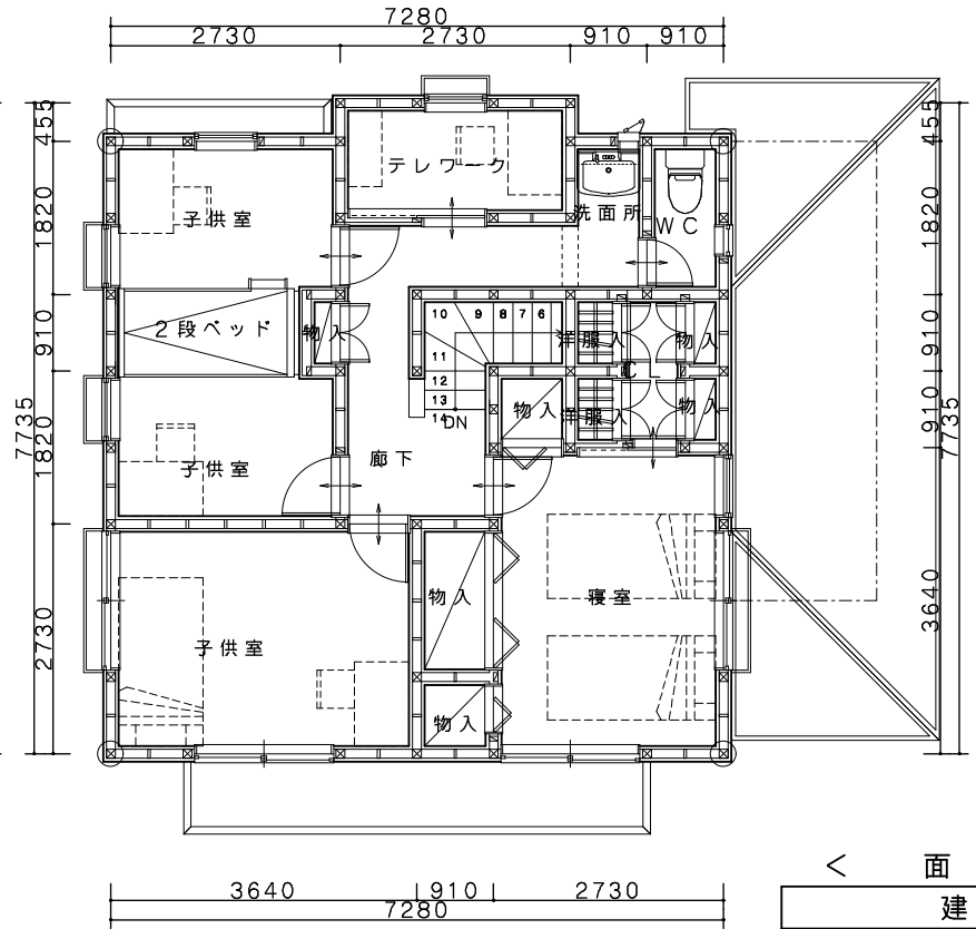
2階平面図
