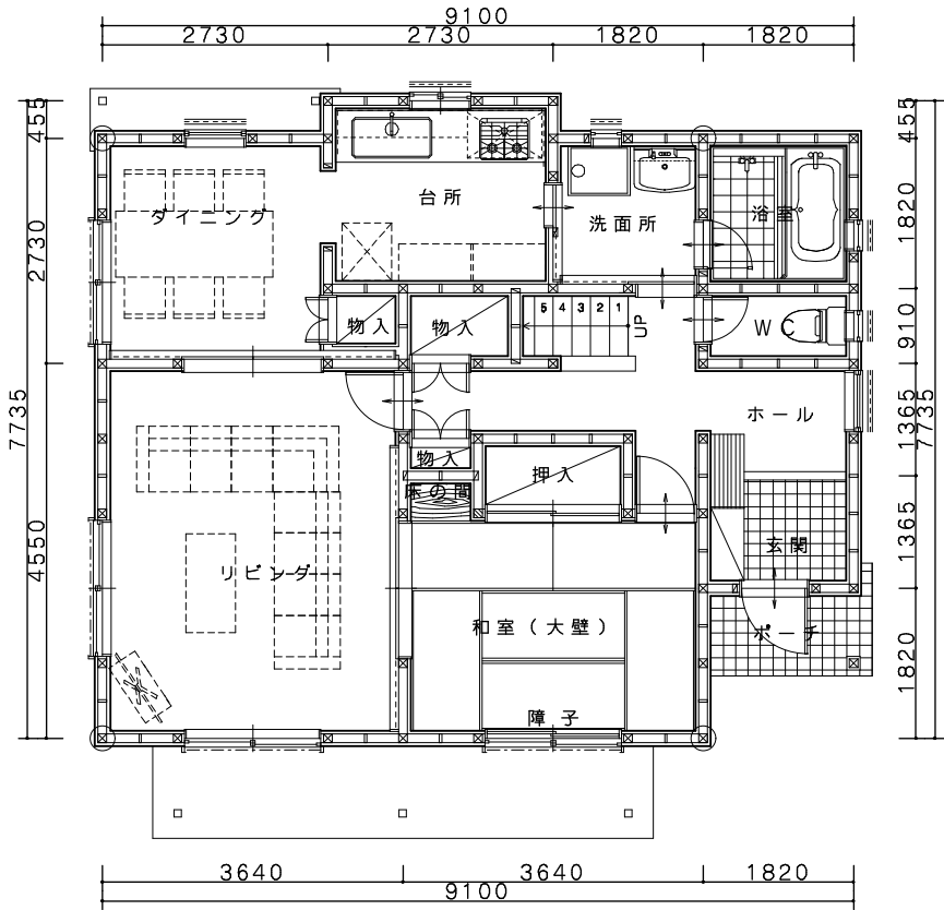
1階平面図
