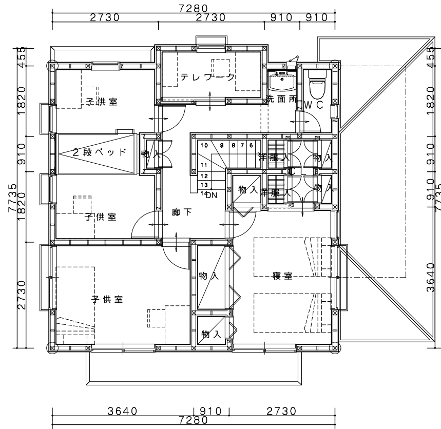
2階平面図
