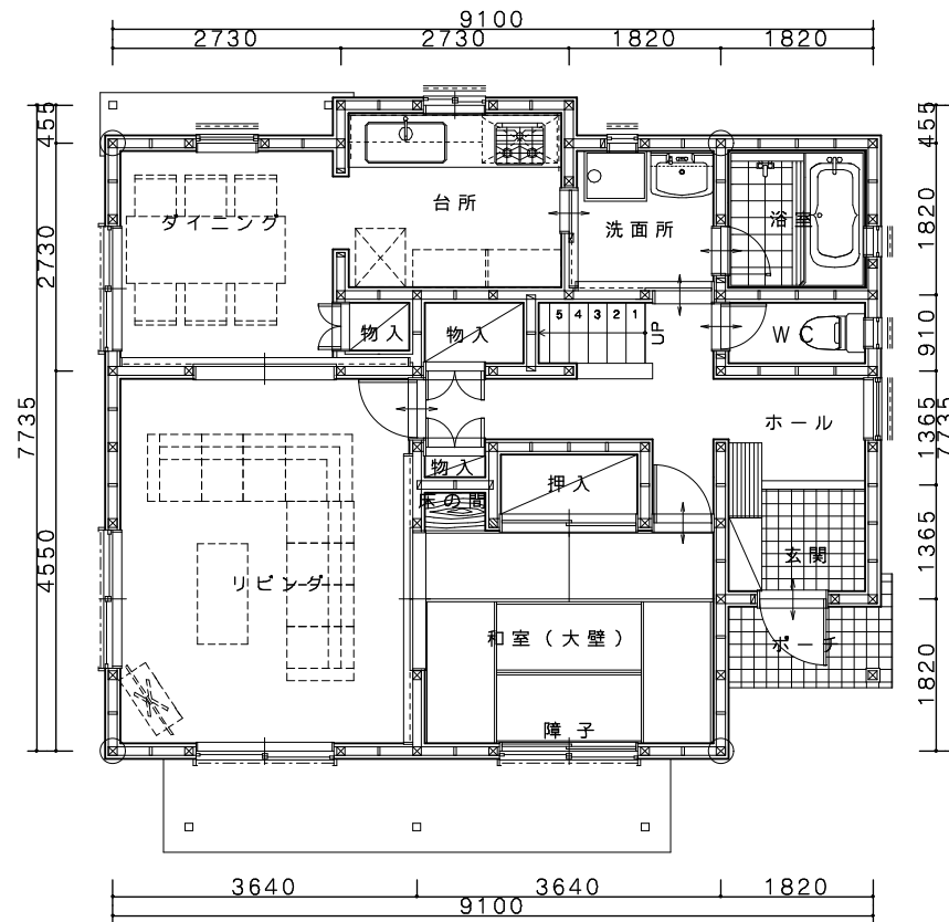
1階平面図
