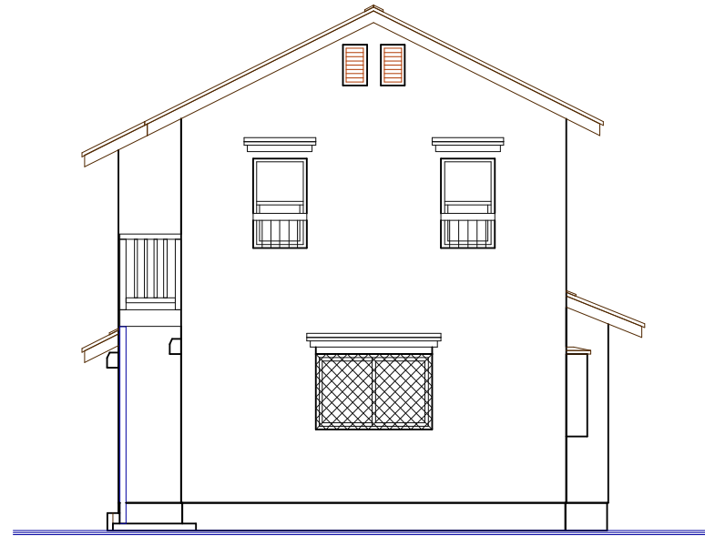
東側立面図
