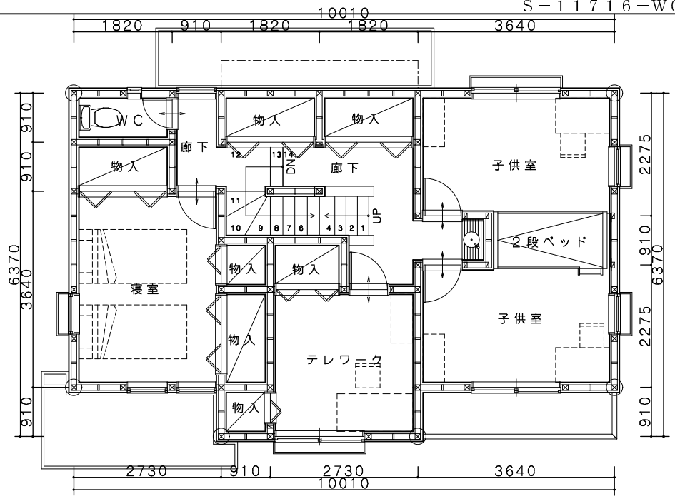
2階平面図
