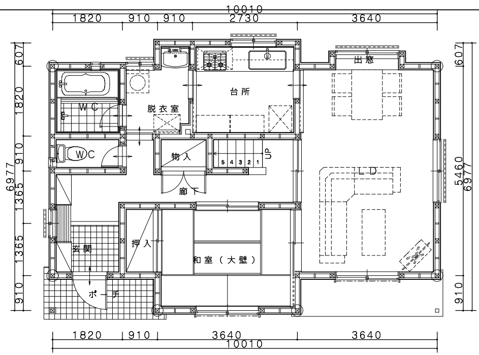
1階平面図
