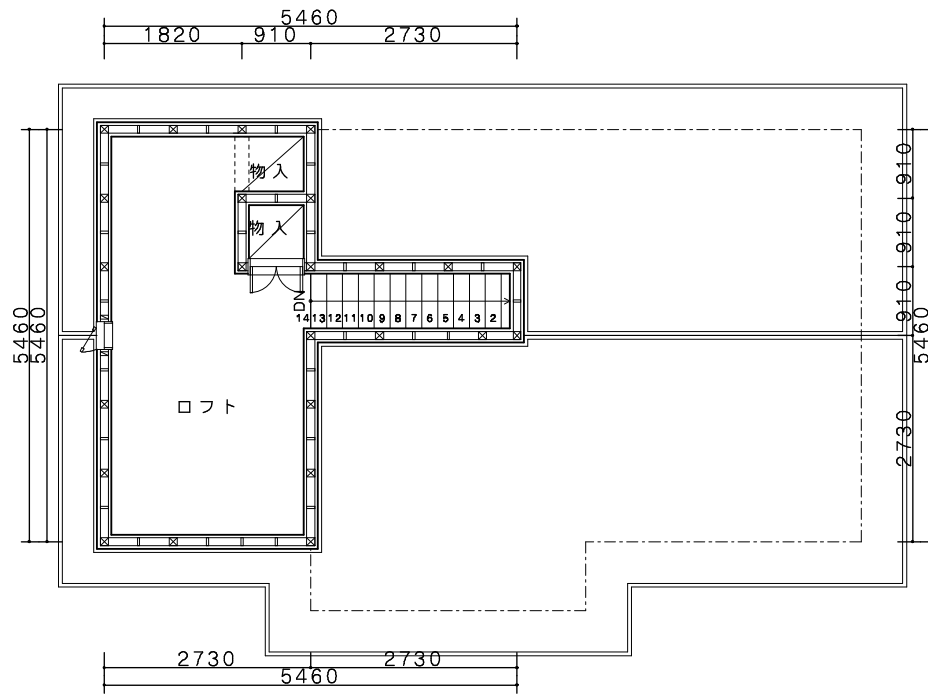
3階平面図
