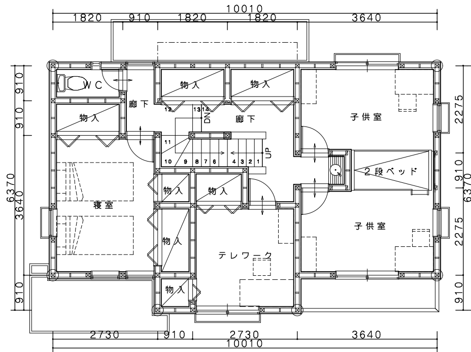
2階平面図
