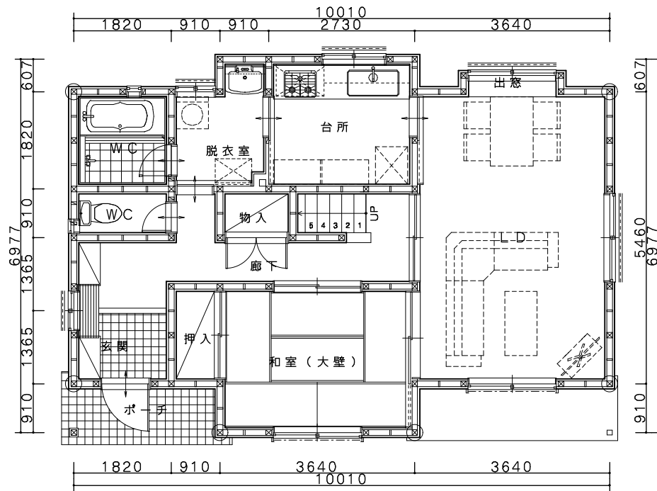
1階平面図
