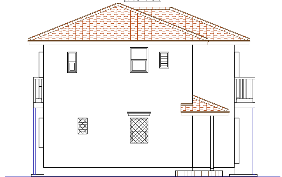
西側立面図
