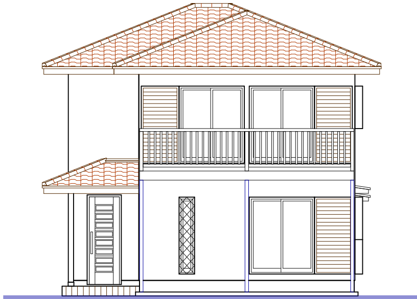
南側立面図
