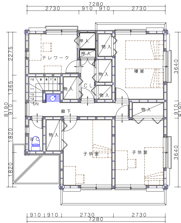
2階平面図
