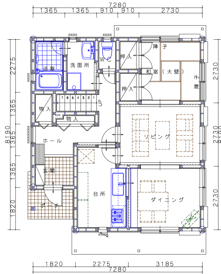
1階平面図
