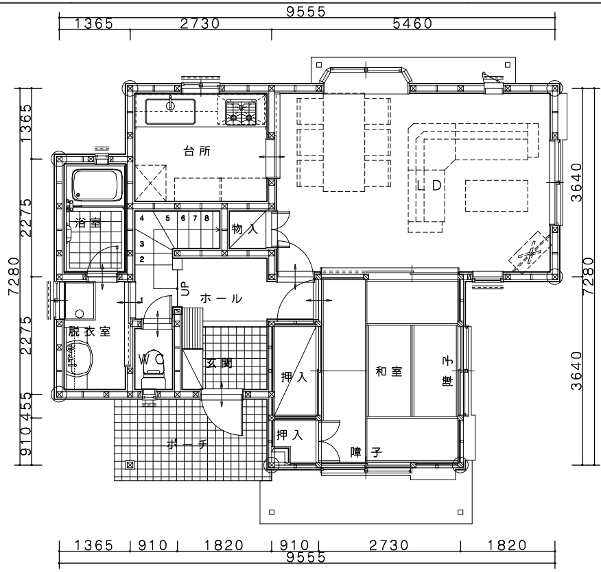
1階平面図
