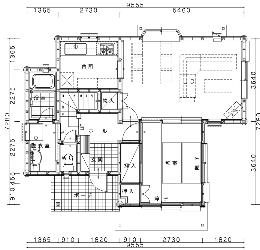
1階平面図
