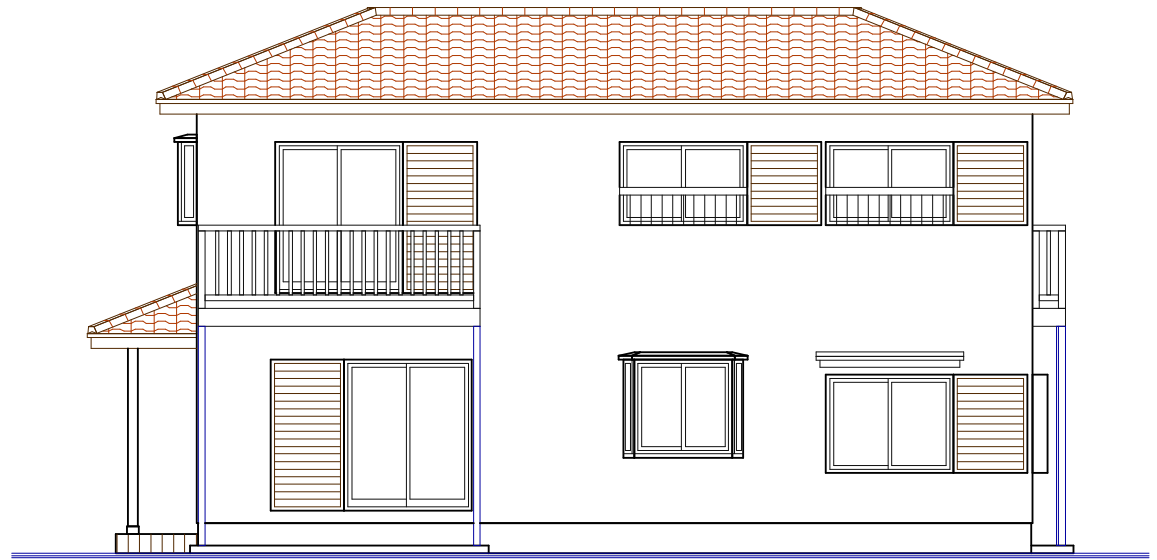
東側立面図
