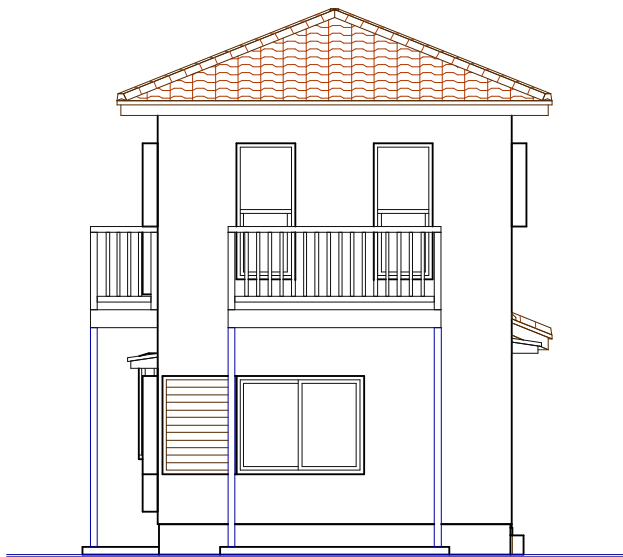
北側立面図
