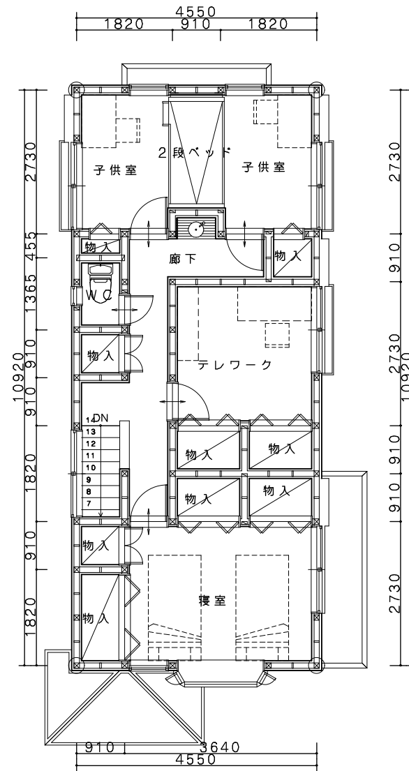
2階平面図
