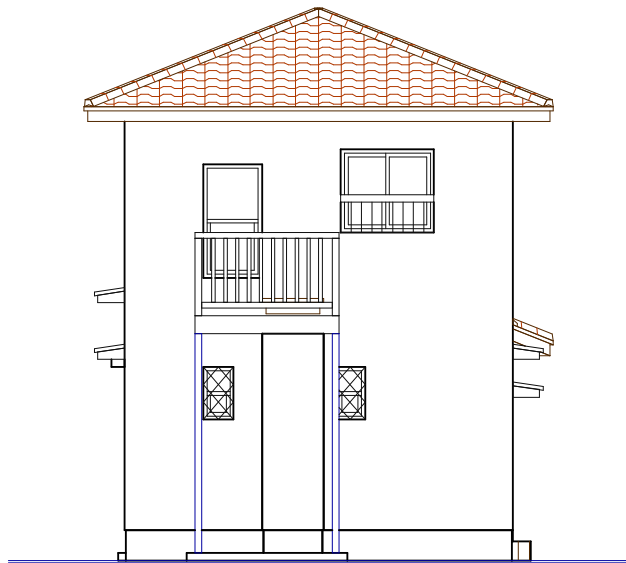
北側立面図
