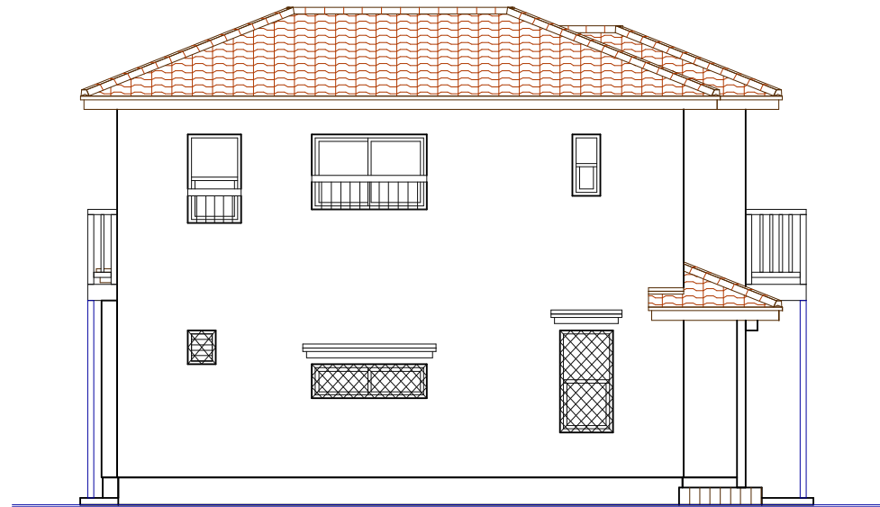
西側立面図
