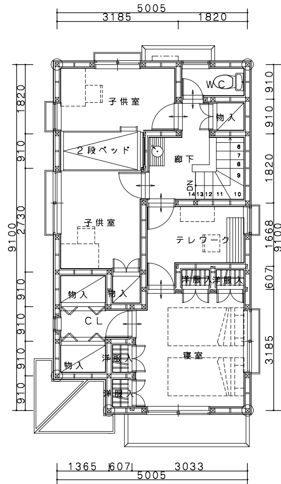
2階平面図
