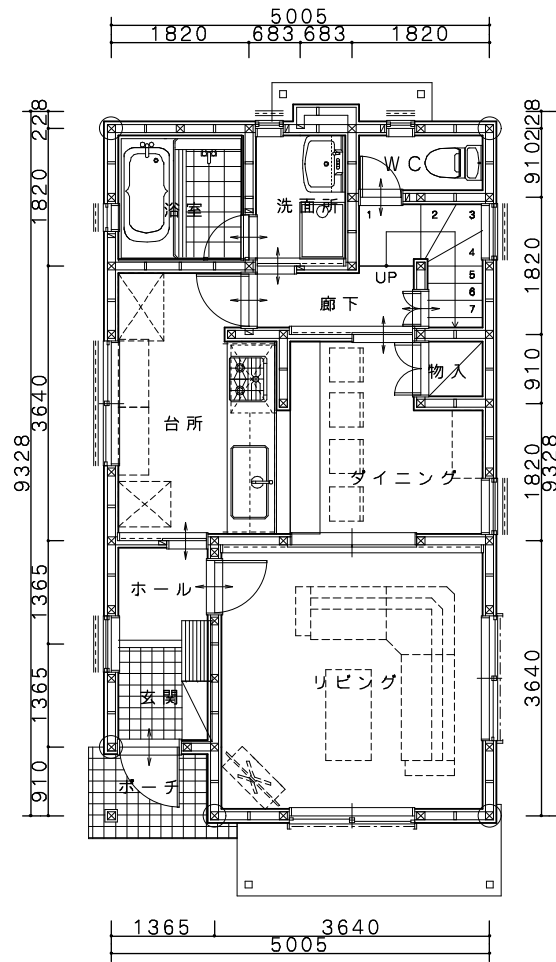
1階平面図
