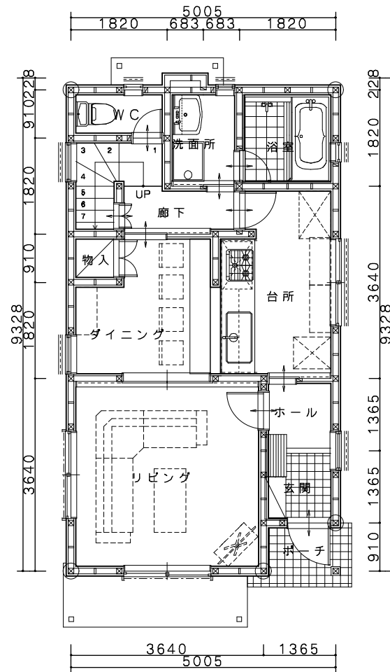
1階平面図
