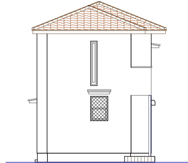
西側立面図
