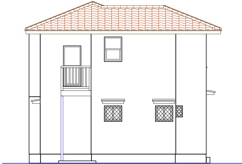
北側立面図
