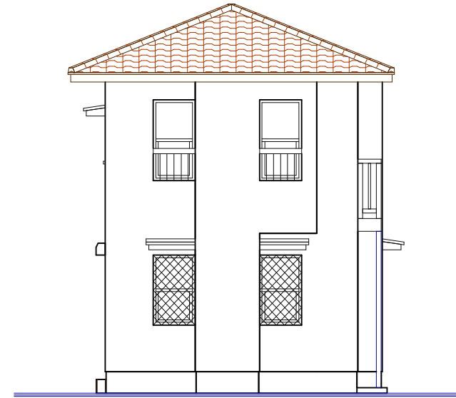
東側立面図
